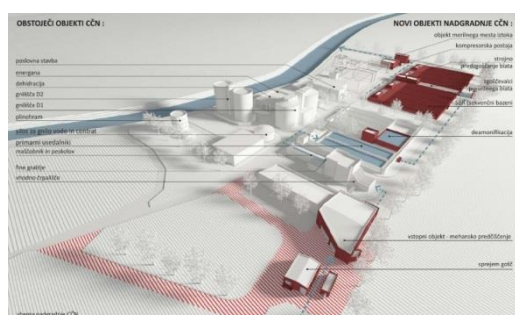
Shema nadgrajene CČN z obstoječimi in novimi procesnimi sklopi
